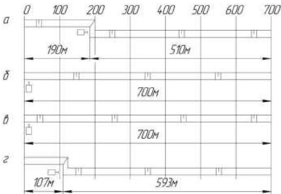
Рис. 2. Ескізи розташування екскаваторного вибою
