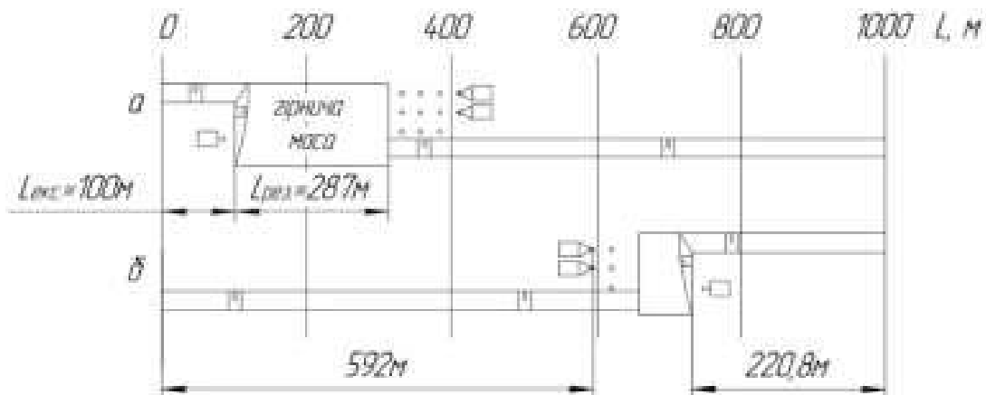
Рис. 6. Розташування мехлопати і бурових верстатів на уступі:
