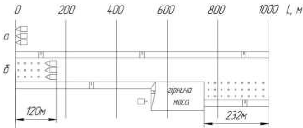
Рис. 4. Розташування бурових верстатів на уступі:
