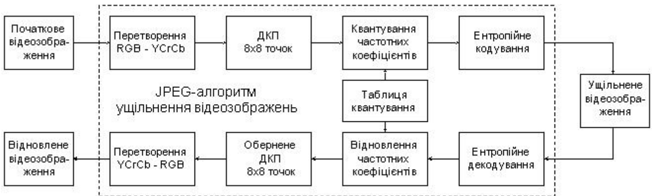
Рис. 2.1. Схема JPEG-алгоритму стиснення цифрових відеозображень
