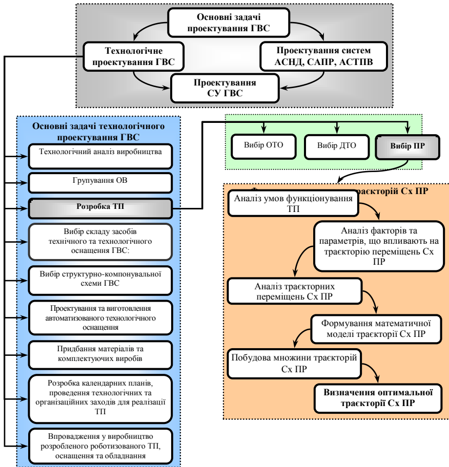
Рис. 13.1. Зміст та місце задачі формування оптимальної траєкторії СхПР та РМСТ при проектуванні ГКС
