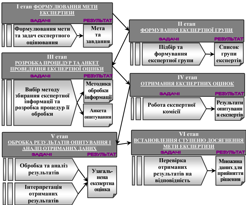
Рис. 13.1. Технологія проведення експертного оцінювання
