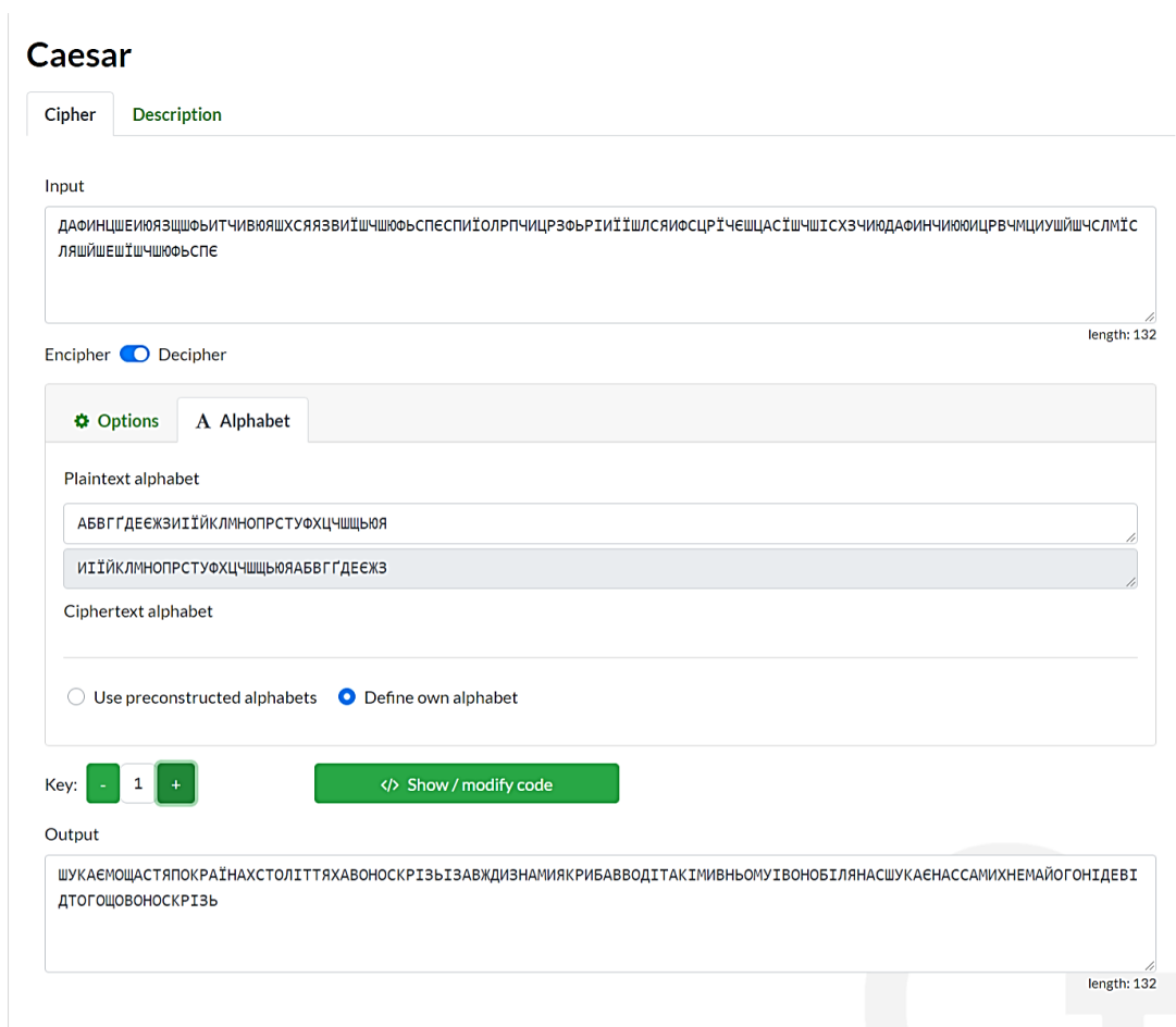
Рис. 1.6. Спроба відновлення повідомлення з підбраним ключем
